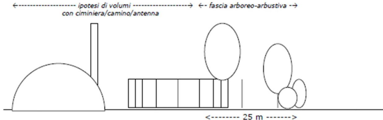
Schema profilo di impianto biomassa o biogas
